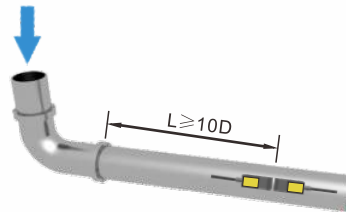
90° Bend
